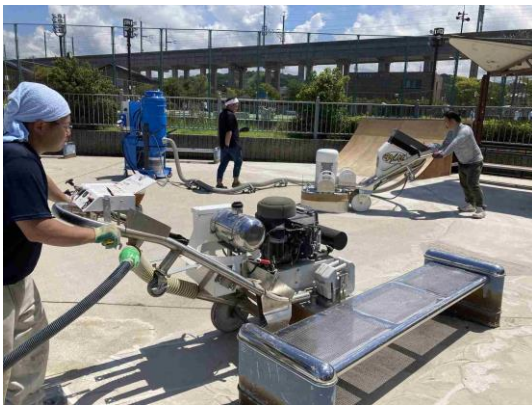
施工風景
